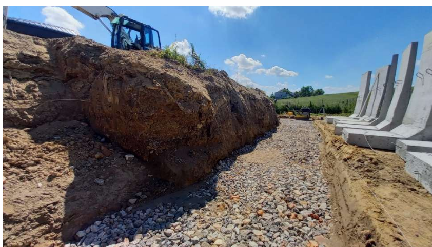
Rys. 3b. Warstwa podbudowy z kruszywa
