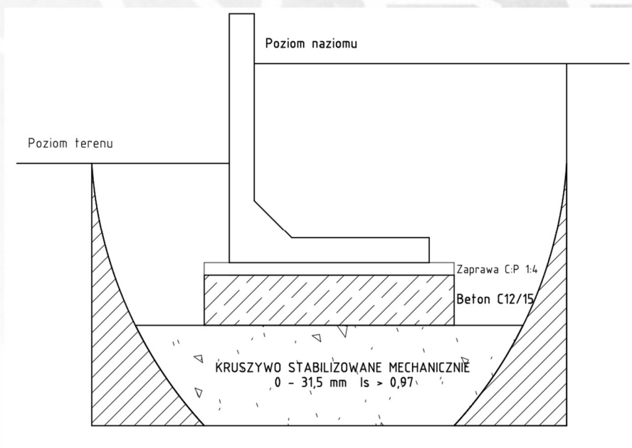
Rys. 3a. Ogólne wytyczne instalacji murów oporowych.
