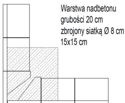
Rys.8.Schemat wykonania narożnika z warstwą nadbetonu.
