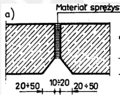
Rys.5. Szczegóły wypełnienia przerwy konstrukcyjnej i dylatacyjnej między prefabrykatami.
